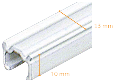
Riel barras (6 mts.)
