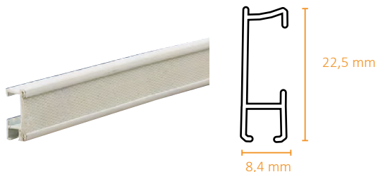
Perfil stor (6 m.)*
